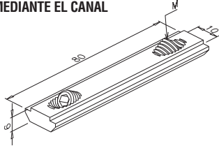
PLETINA PARA UNIR PERFILES MEDIANTE EL CANAL
