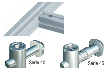
CONECTOR DE PERFILES "ALUSKIT®" CABEZA REDONDA
