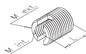
CASQUILLO REDUCTOR
