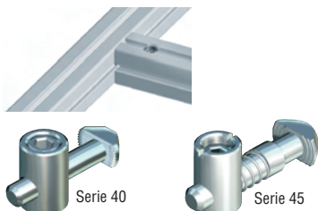
CONECTOR DE PERFILES "ALUSKIT®" PERPENDICULAR
