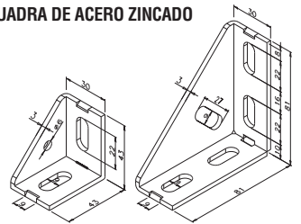
ESCUADRA DE ACERO ZINCADO
