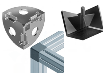
ESQUINERO Y TAPA CON ARISTA VIVA S30
