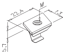
TUERCA ROMBO CON MUELLE
