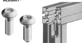
TORNILLOS PARA ENSAMBLAR PERFILES "ALUSKIT®"
