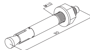
TACO DE EXPANSIÓN PARA ANCLAJE A SUELO
