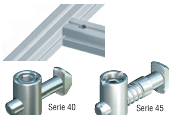
CONECTOR DE PERFILES "ALUSKIT®" PARALELO
