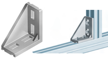
ESCUADRA DE ALUMINIO INYECTADO 57 x 57 x 28 mm.
