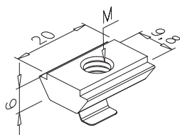
TUERCA RECTANGULAR CON MUELLE
