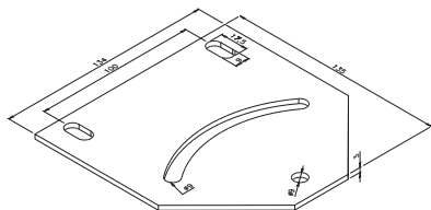
PLACA COMPÁS PLANA GIRATORIA
