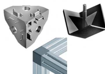
ESQUINERO Y TAPA CON ARISTA VIVA S40
