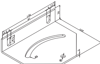
PLACA COMPÁS ANGULAR GIRATORIA
