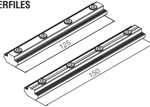
REGLETA DE UNION DE PERFILES
