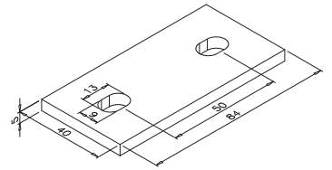
PLETINA PARA UNIR PERFILES
