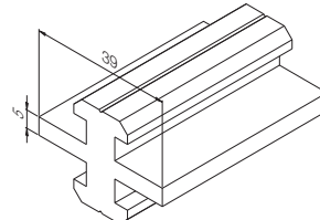
GUIA DESLIZANTE DOBLE
