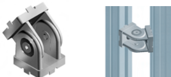
ARTICULACIÓN GRADUABLE 30 x 30 CANAL DE 8 mm.
