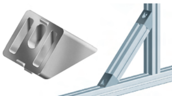
ESCUADRA CONEXIÓN FIJA A 45° S PARA PERFIL DE 40 x 40 mm.
