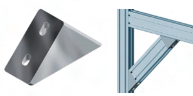
ESCUADRA CONEXIÓN FIJA A 45° S PARA PERFIL DE 80 x 80 mm.
