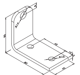
ÁNGULO DE SUJECIÓN
