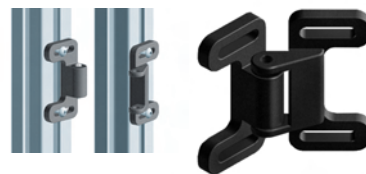
BISAGRA-FIJADOR DE MARCOS
