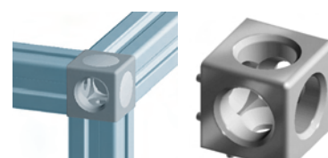
CUBO ENSAMBLE A TRES VIAS "ALUSKIT®"
