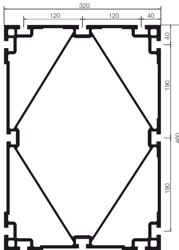
140306 PERFIL 460x320 LIGERO
