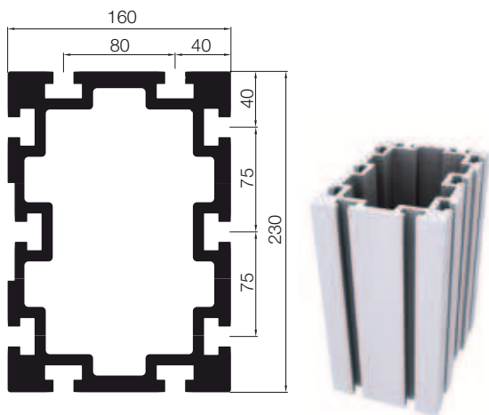
140303 PERFIL 230x160 REFORZADO
