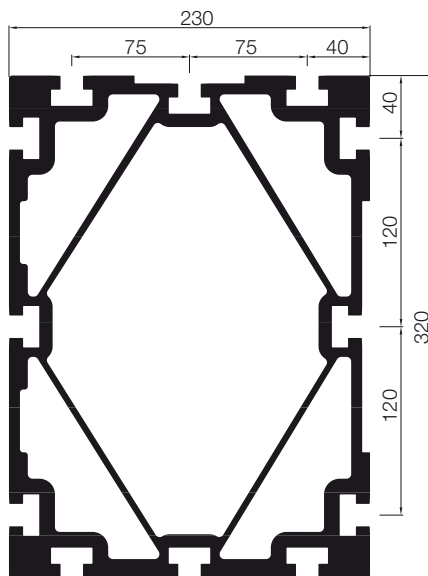
140305 PERFIL 160x115 REFORZADO
