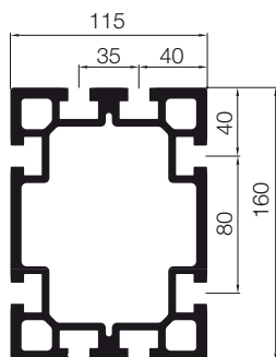
140301 PERFIL 160x115 LIGERO
