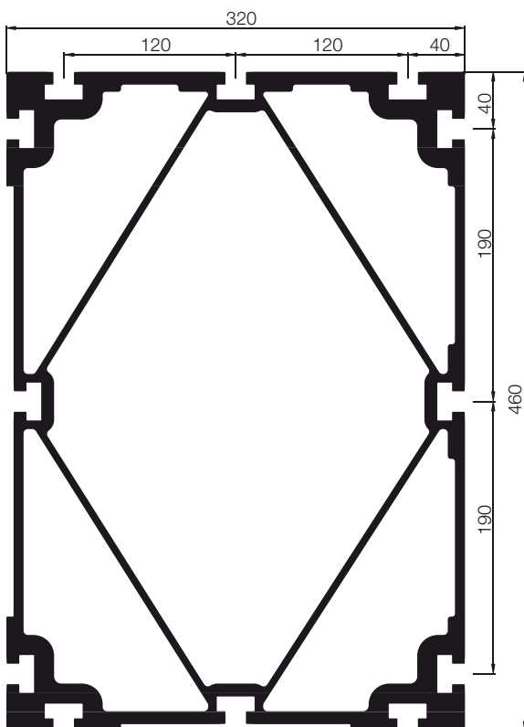
140307 PERFIL 320x230 REFORZADO
