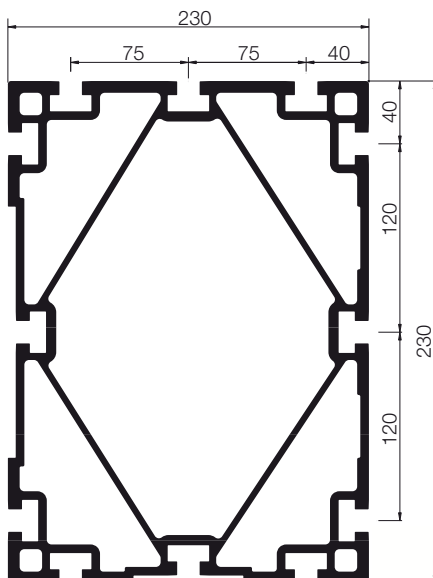
140304 PERFIL 320x230 LIGERO
