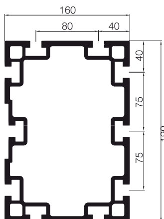
140302 PERFIL 230x160 LIGERO
