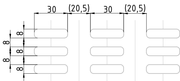
DETALLE PERFORACIÓN - ÁREA PERFORADA 28,7%
