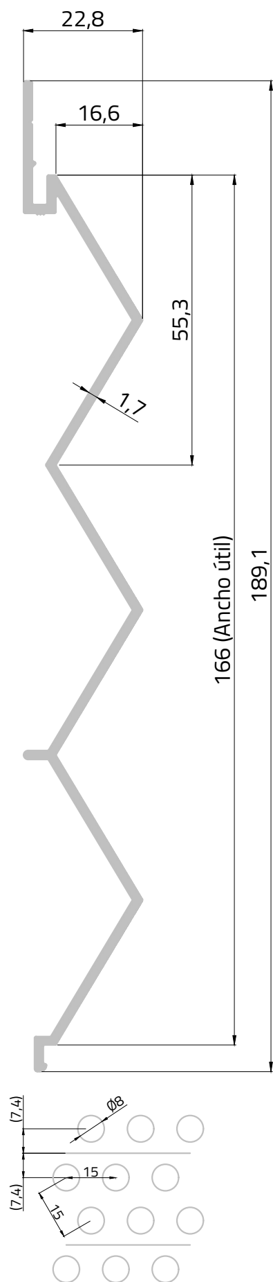
DETALLE PERFORACIÓN - ÁREA PERFORADA 20,2%
