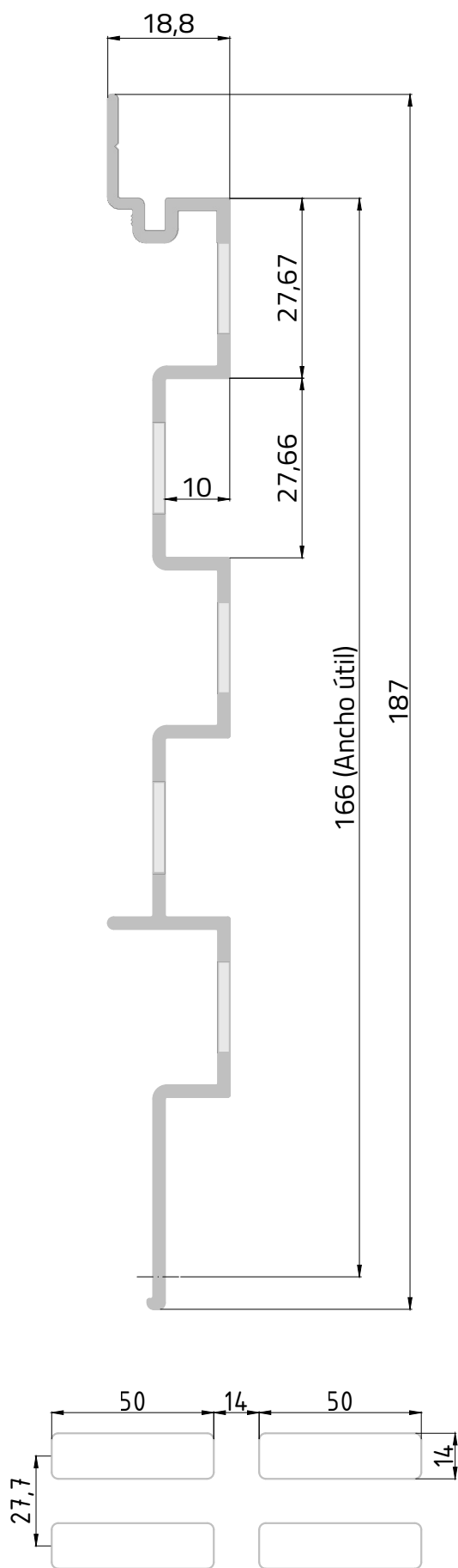
DETALLE PERFORACIÓN - ÁREA PERFORADA 32,7%
